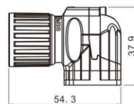
Розетка на панель, угловая
