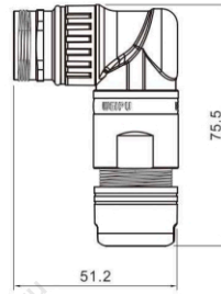
Вилка кабельная, угловая
